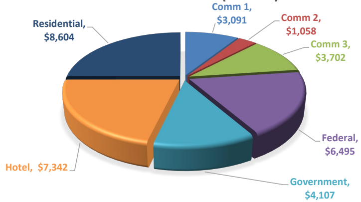
in mGals
